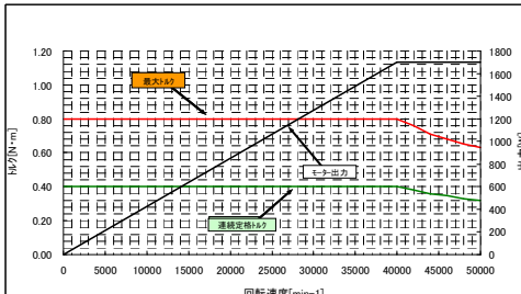
DL56CT トルク特性
