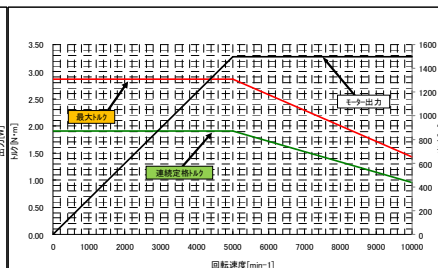
DL120 トルク特性
