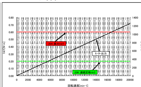
20K トルク特性
