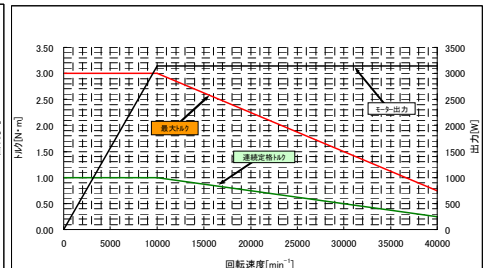
DL68CT トルク特性
