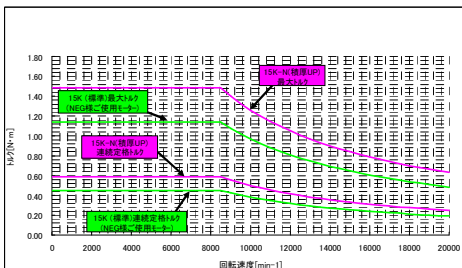
DL5440 トルク特性
