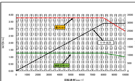
DL8282 トルク特性
