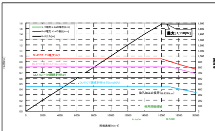
DL47CT トルク特性
