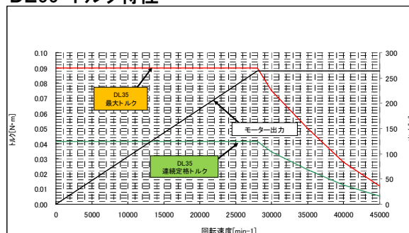
DL35 トルク特性
