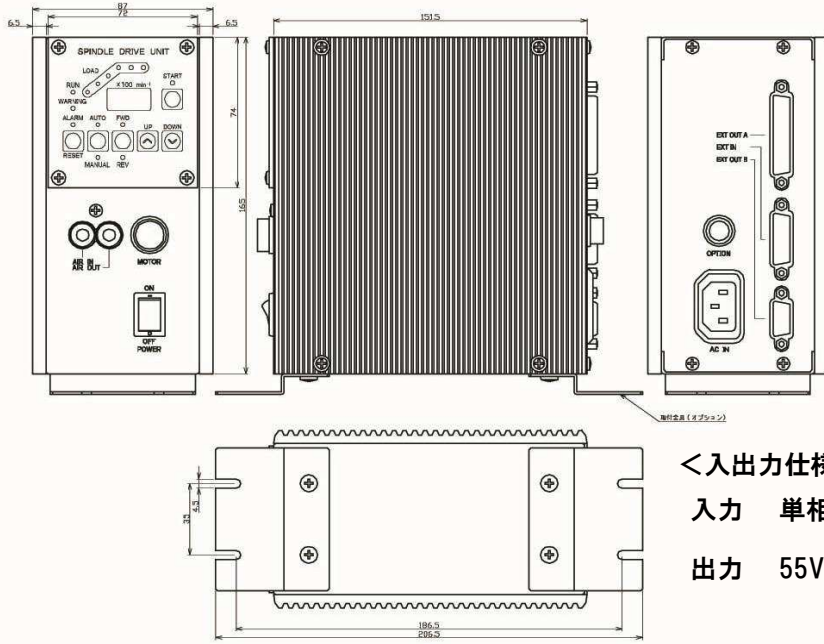
重量:2.5kgtyp
