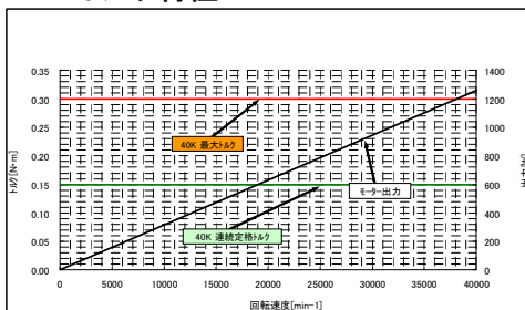
40K トルク特性
