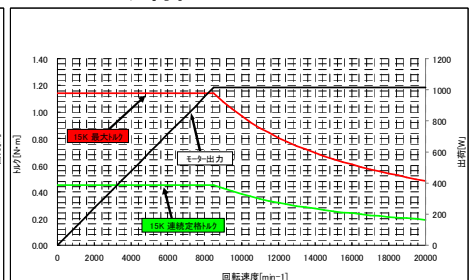
15K トルク特性
