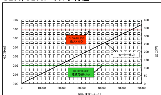
DL30/DL30F トルク特性
